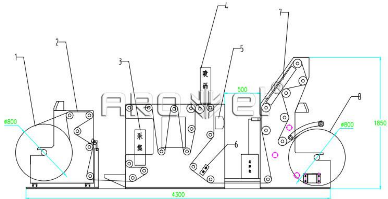
1. 放卷 2. 电晕机位 3. 采集检测位 4. 喷码 5. UV 6. 检测 7. 频闪观测位 8. 收卷
